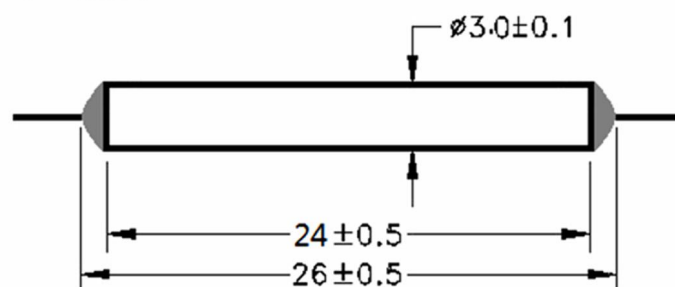
Mini光纤隔离器
