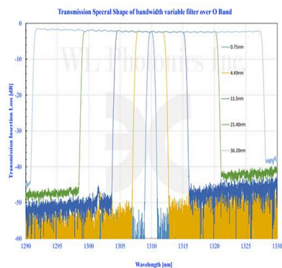
P型带宽可调谐滤波器在O波段的传输光谱
