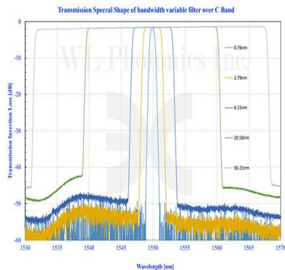
P型带宽可调谐滤波器在C波段的传输光谱
