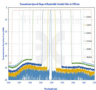
U型带宽可调谐滤波器在C波段的传输光谱
