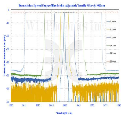
U型带宽可调谐滤波器在X波段的传输光谱
