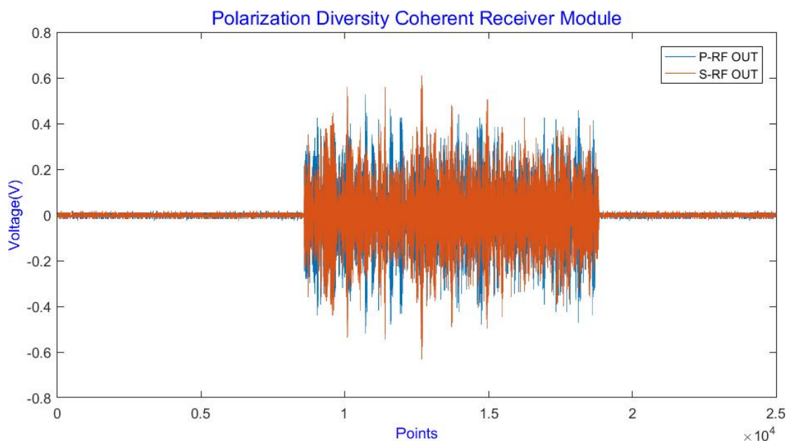
P 偏振态和 S 偏振态相干信号
