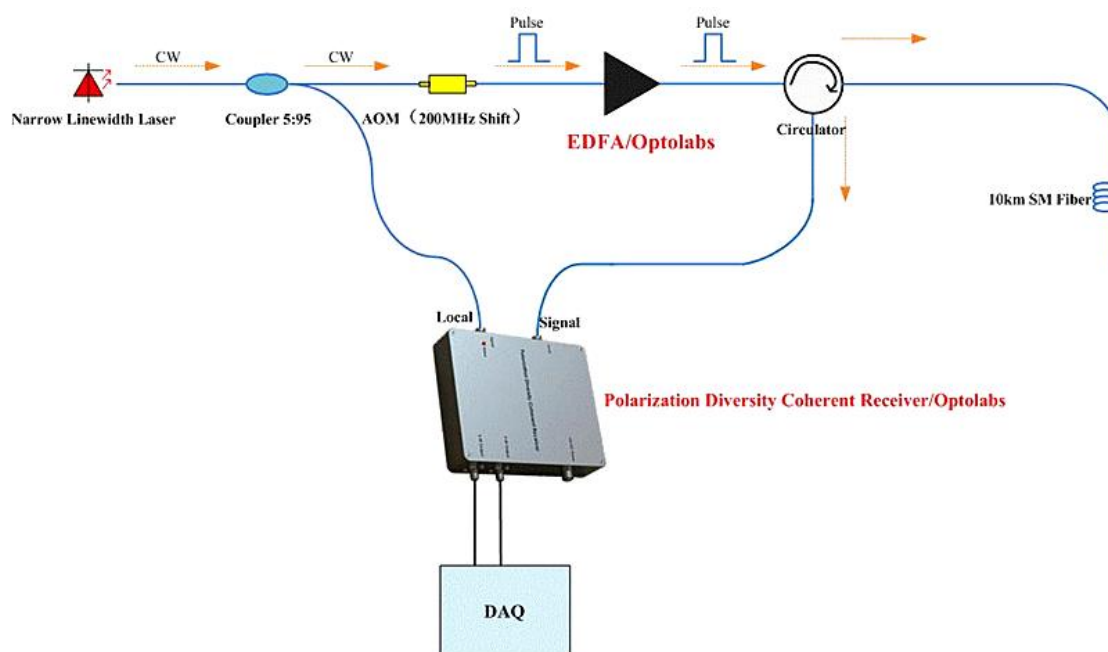
偏振分集相干接收光路图
